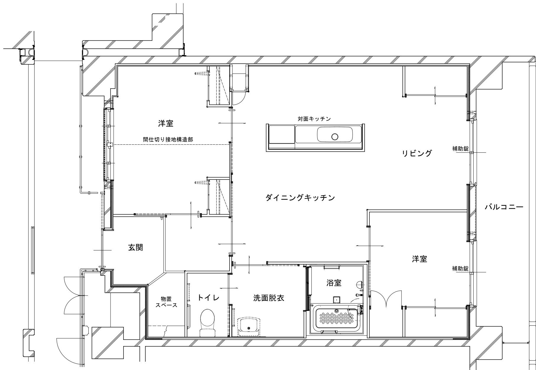
県営西玉江団地子育て支援住宅平面図
