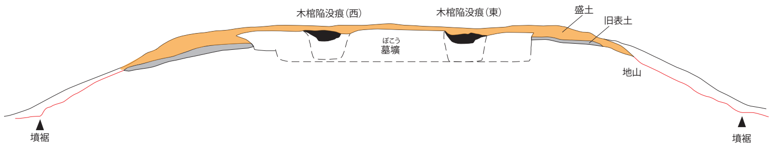
名分丸山1号墳後方部墳丘横断面模式図
