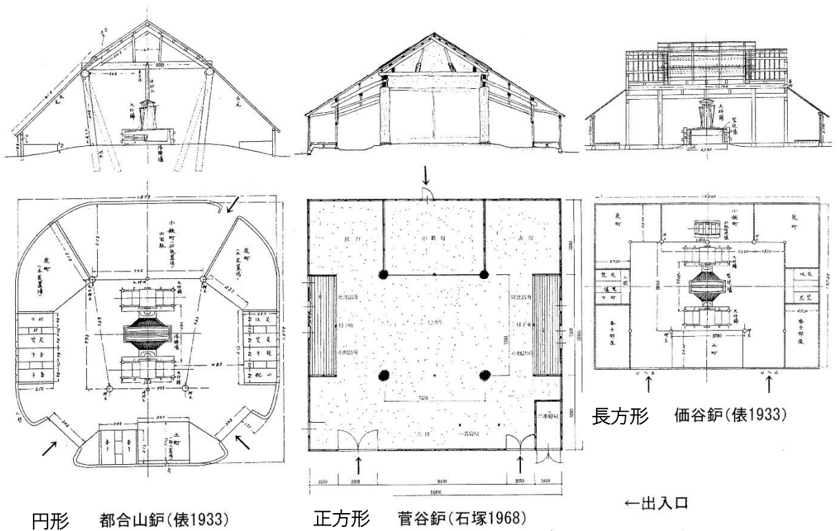
高殿の3類型 角田徳幸 2014 「たたら吹き製鉄の成立と展開」より転載 (一部改変)
