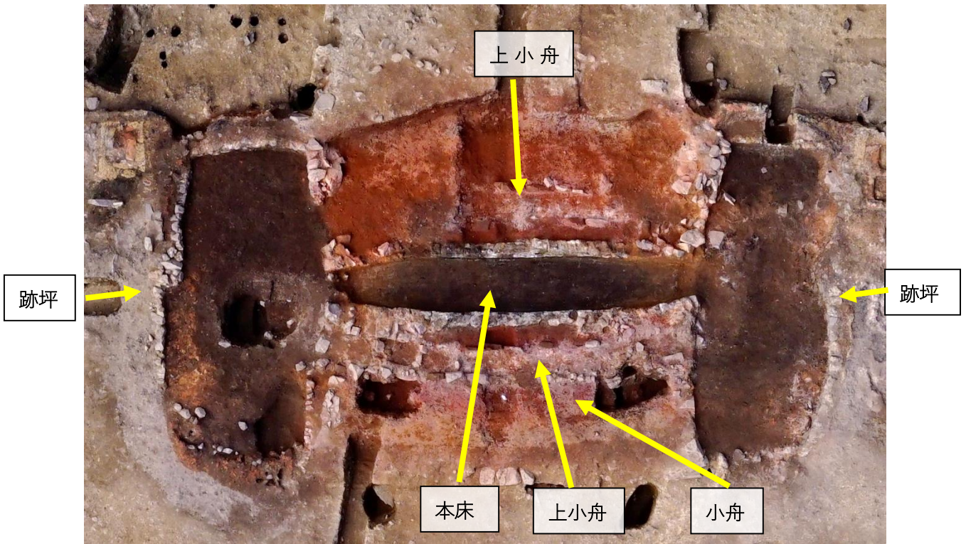
桜谷鉦跡 製鉄炉地下構造
