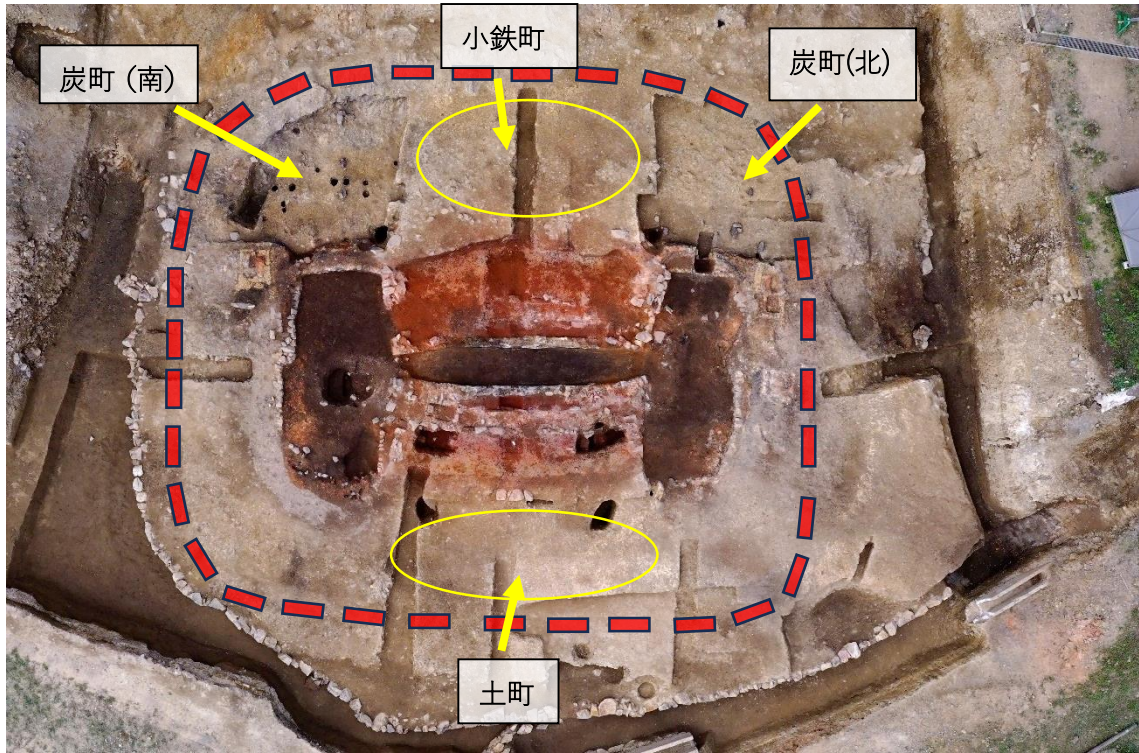
桜谷鉦跡 高殿内の主要遺構 点線は高殿の推定輪郭線
