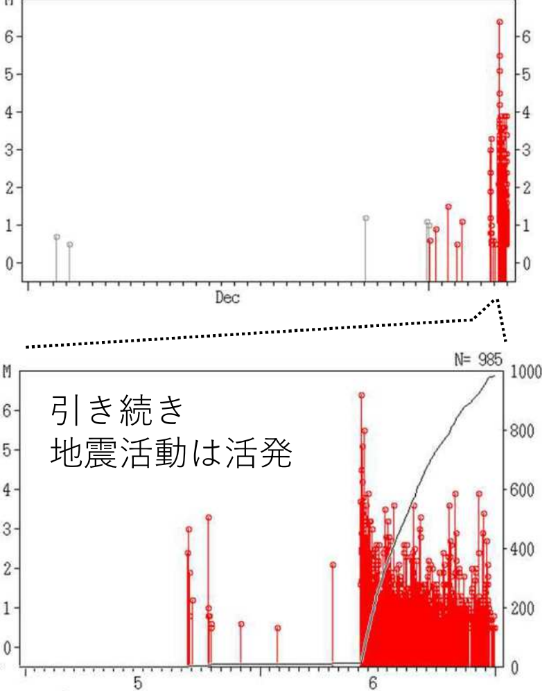
【左図の青色四角形領域内の地震活動経過図】
