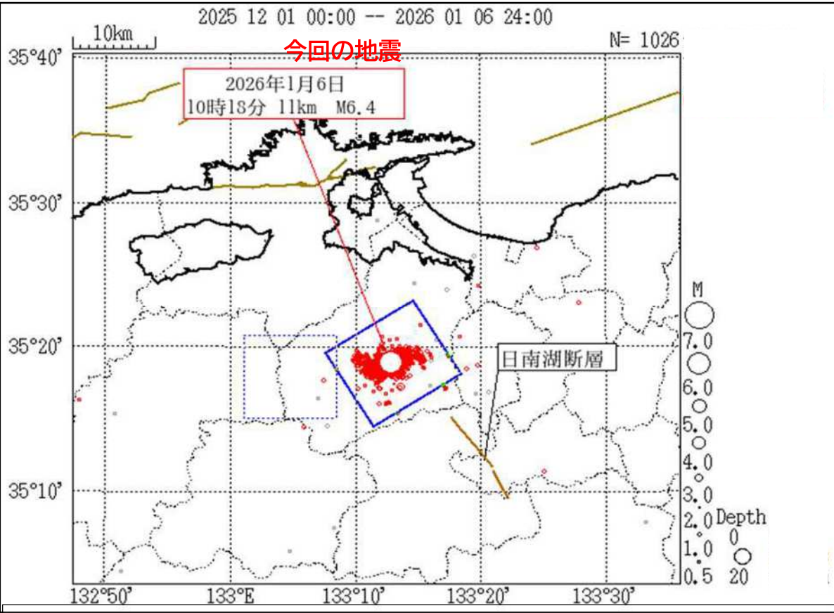
【震央分布図】 (2025年12月1日～2026年1月6日24時、深さ0～20km、 M \geq 0.5 ) 丸の大きさはマグニチュードの大きさを表示 地震調査研究推進本部の長期評価による活断層を細線で表示
