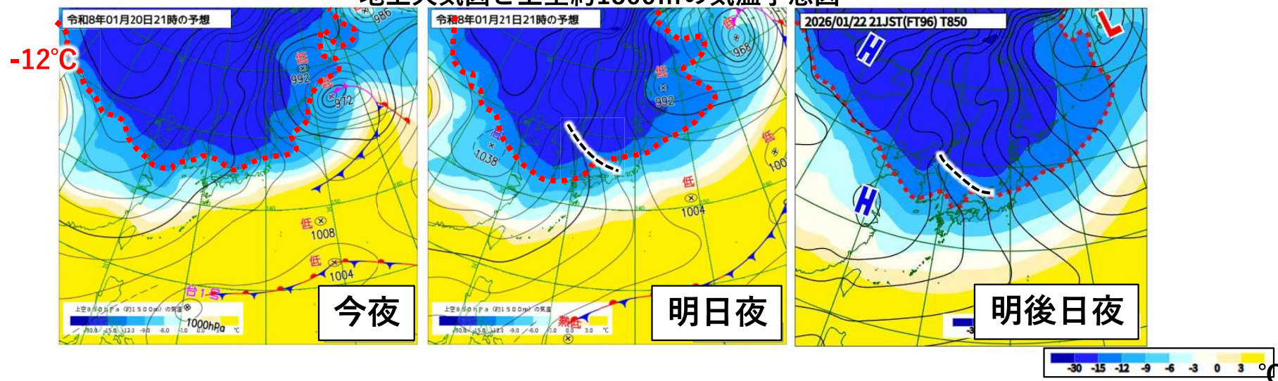
地上天気図と上空約1500mの気温予想図
