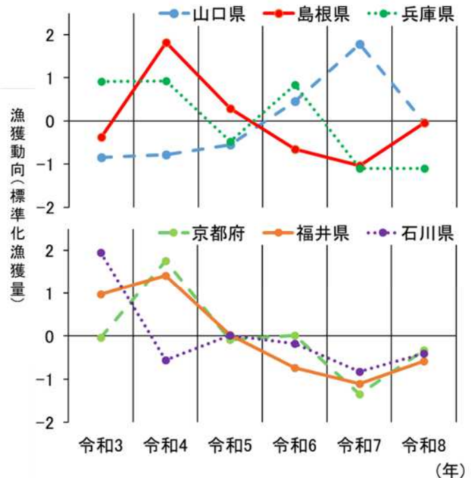
図2. 日本海西部各府県のトビウオ類の漁獲動向（標準化漁獲量） 標準化漁獲量：同じ条件で比較するために漁獲量データに統計処理を施したもの
