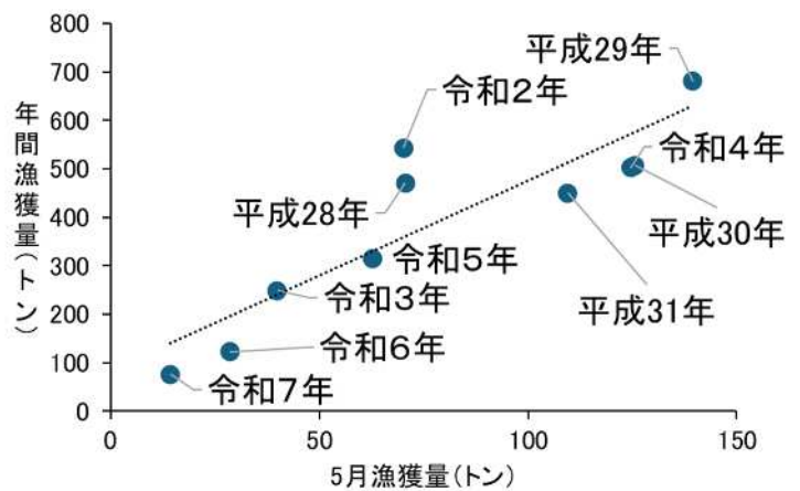
図3. 島根県におけるトビウオ類の5月の漁獲量と年間漁獲量の関係（全漁法）
